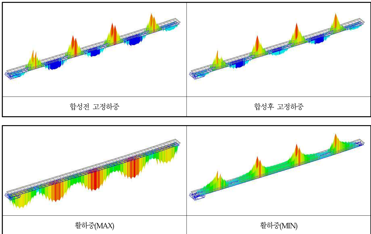
【그림 5.2.19】 휨모멘트도(부산)
