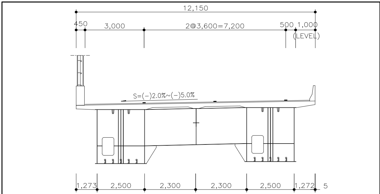
【그림 5.2.1】 해석단면(대구)
