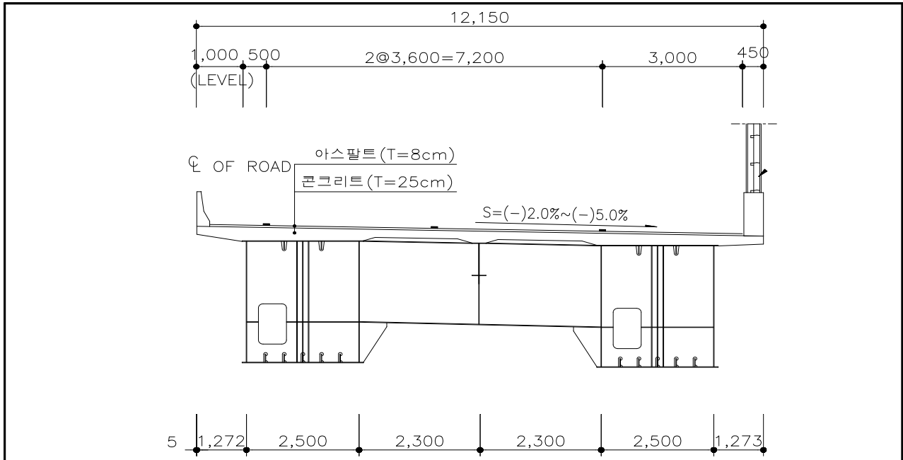
【그림 5.2.13】 해석단면(부산)
