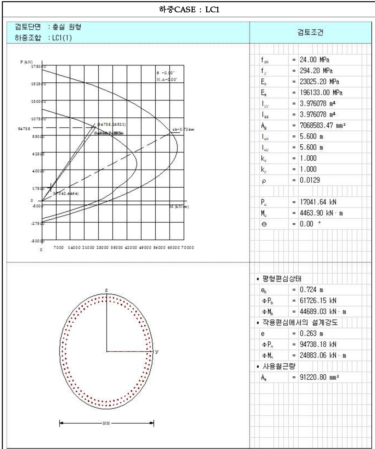
【그림 5.4.14】 P-M 상관도(하중CASE : LC1)(부산)
