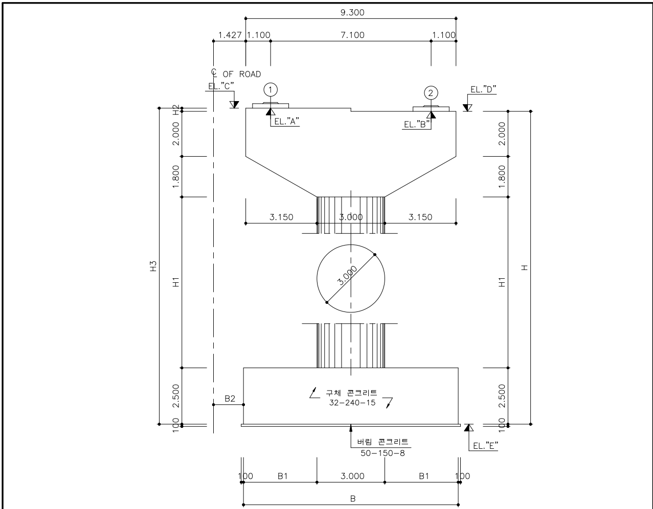
【그림 5.4.12】 해석단면(P3)(부산)
