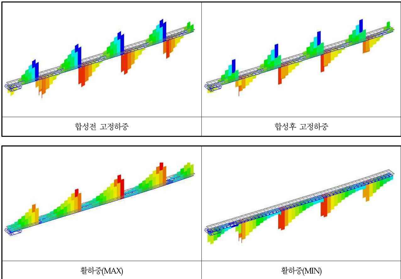
【그림 5.2.20】 전단력도(부산)
